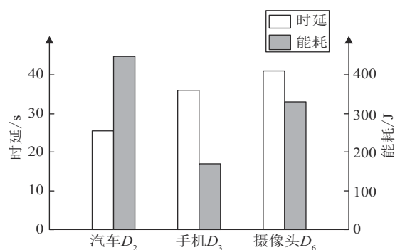
图4 时延和能耗情况仿真结果
