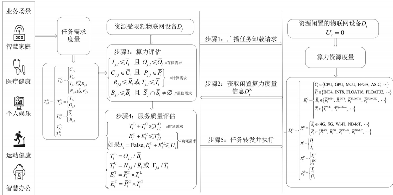
图2 分布式任务调度流程
